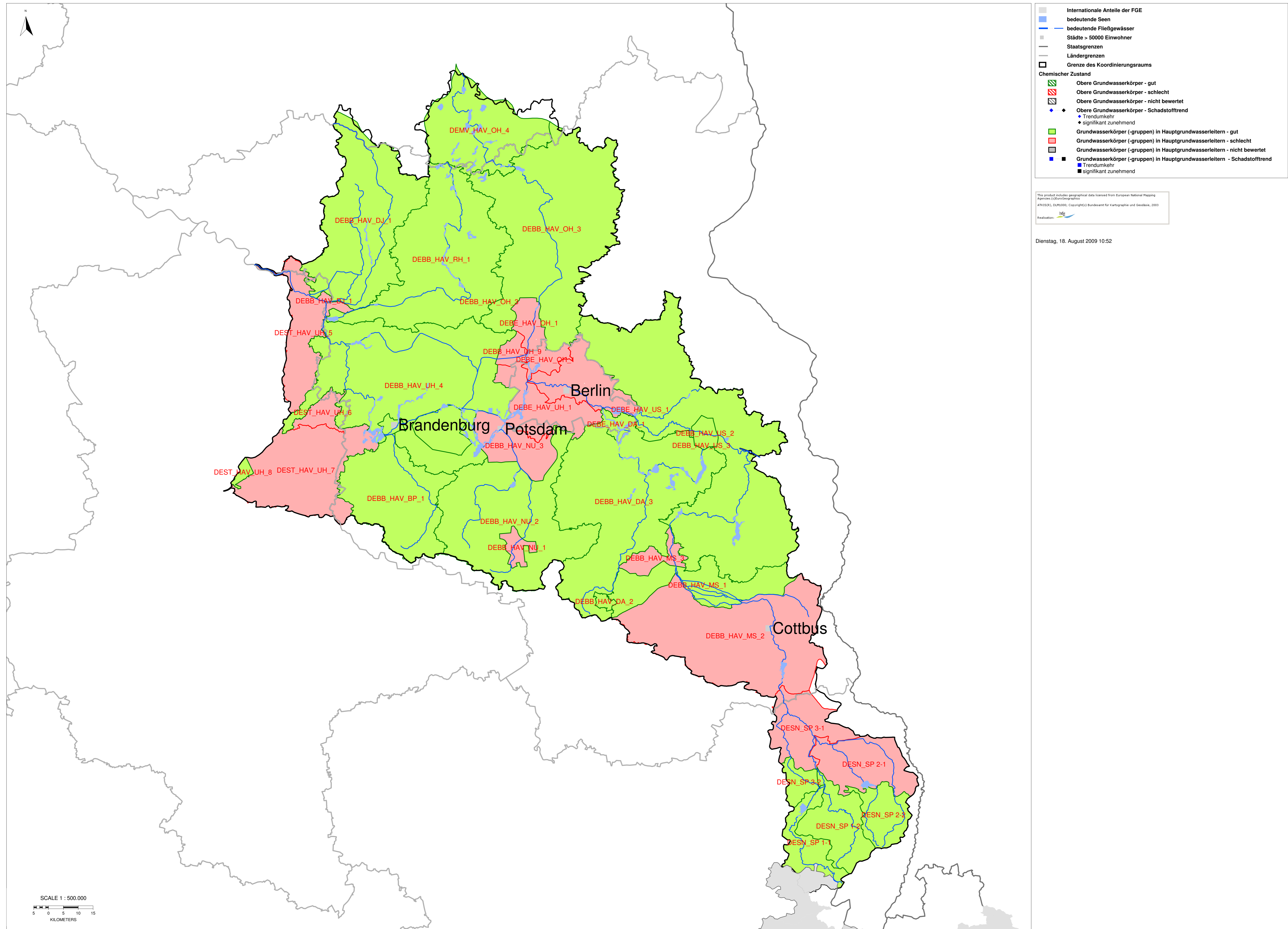
Koordinierungsraum Havel, Karte 4.6: Chemischer Zustand der Grundwasserkörper und Identifikation von Grundwasserkörpern mit signifikant zunehmendem Schadstofftrend
