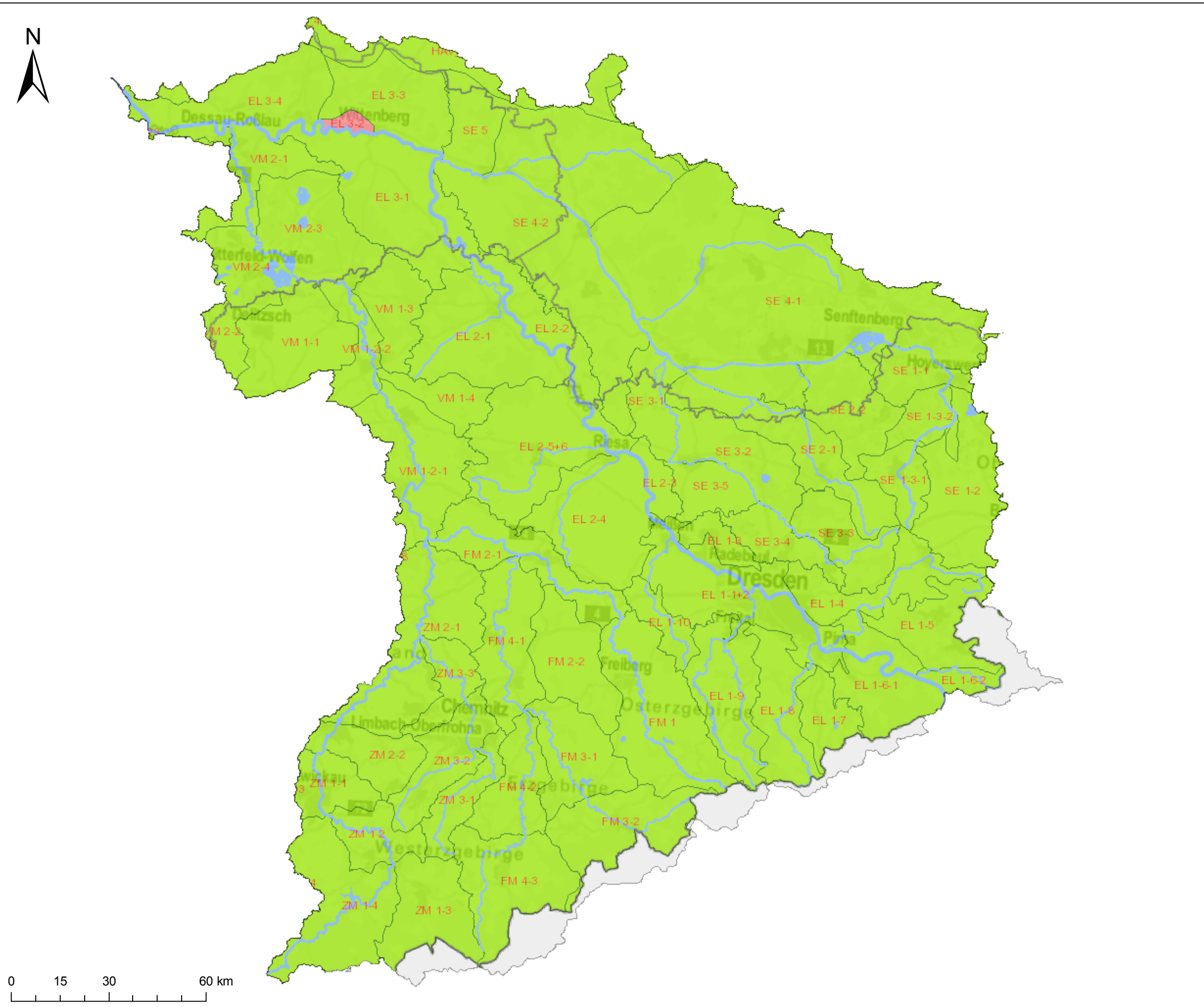
KOR Mulde-Elbe-Schwarze Elster - Karte 4.6.2: Chemischer Zustand der Grundwasserkörper hinsichtlich Pestiziden
